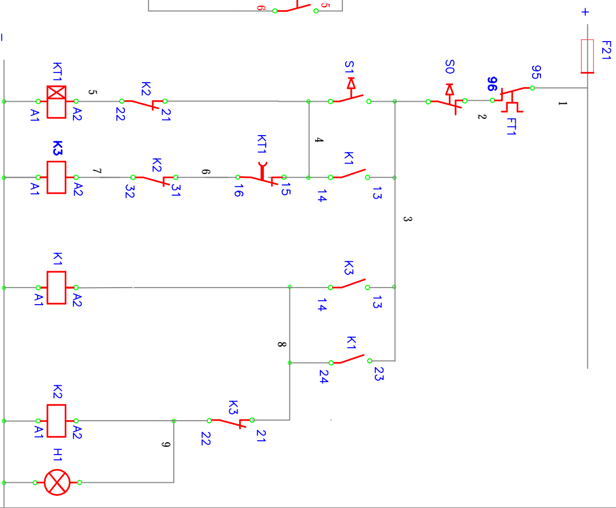
b) Diagrama de comando
